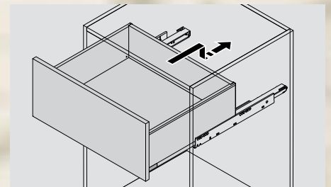
LEGRABOX einhängen
