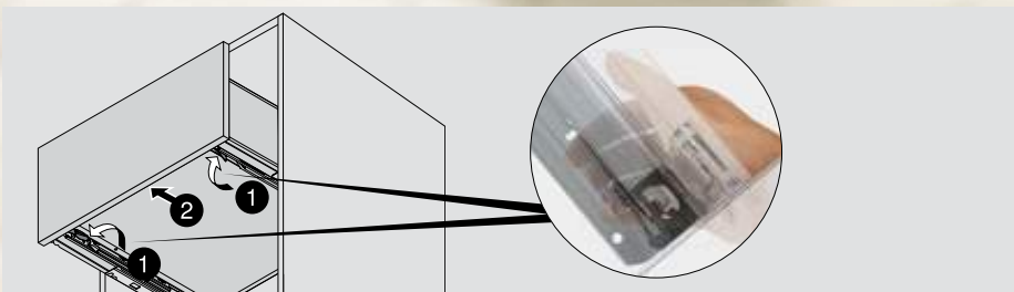
LEGRABOX aushängen (Ansicht von unten)
