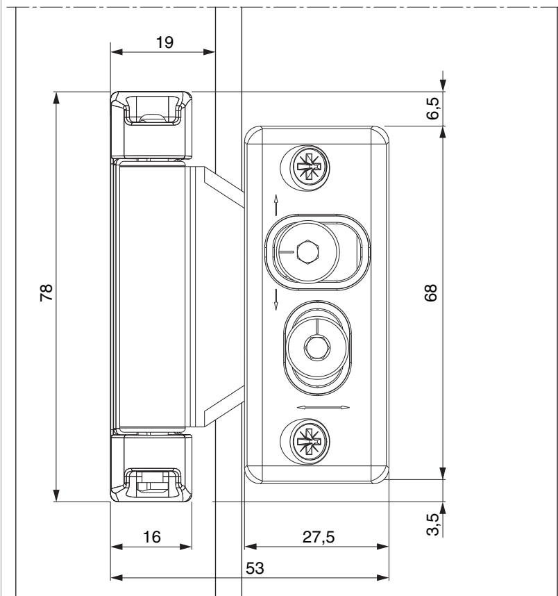
Scherenlager 52480 und Paumellenband Flügelteil 220241 mit Lehre 11888 *
