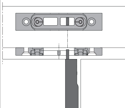
2 flg. Fenster mit 1 Riegel
