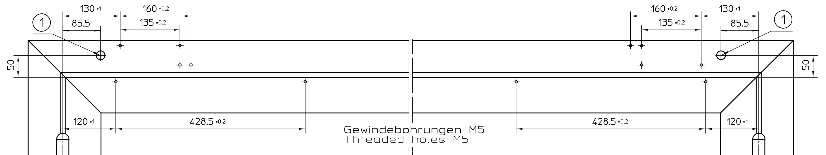
Anschlagmaße für Tür mit Linksflügel Mounting dimensions for door with left leaf
