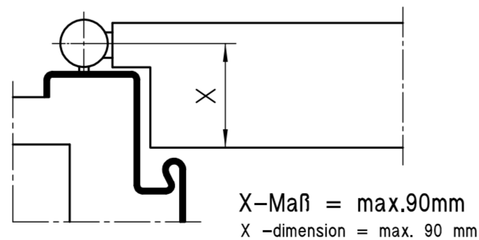
Anschlagmaße für Tür mit Rechtsflügel mounting dimensions for right hand door
