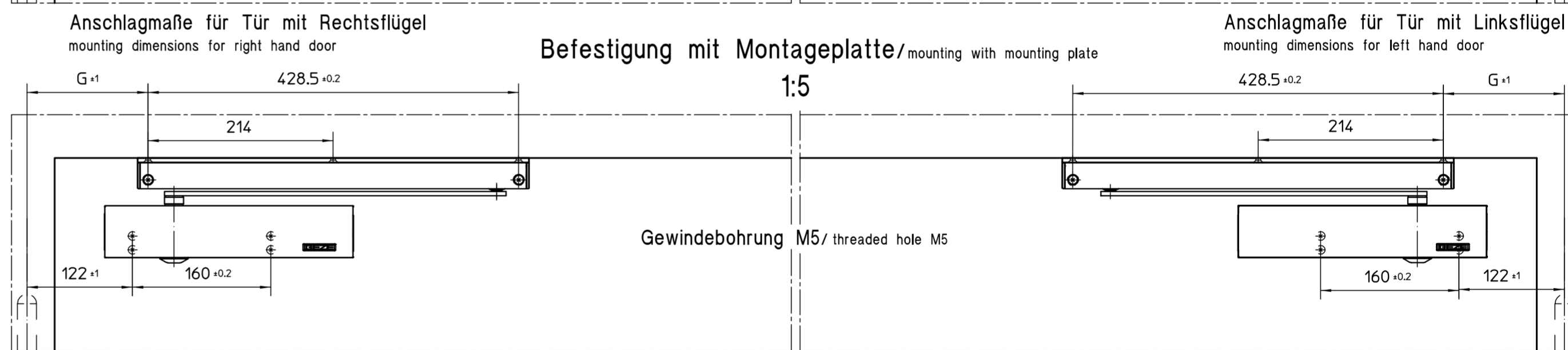
Anschlagmaße für Tür mit Rechtsflügel mounting dimensions for right hand door
