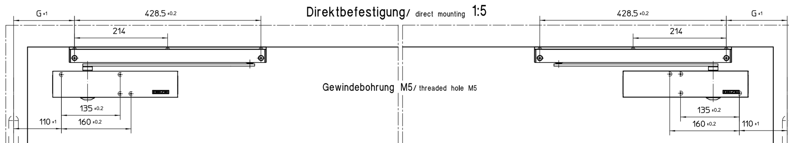
Anschlagmaße für Tür mit Rechtsflügel mounting dimensions for right hand door
