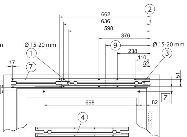
Direktbefestigung
