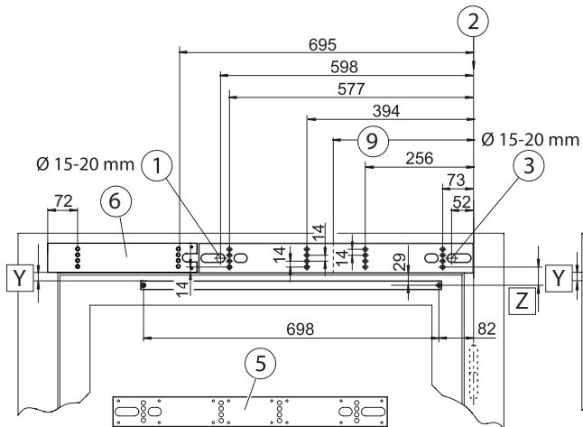
Befestigung mit Montageplatte
