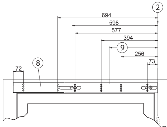
Befestigung mit durchgehender Montageplatte
