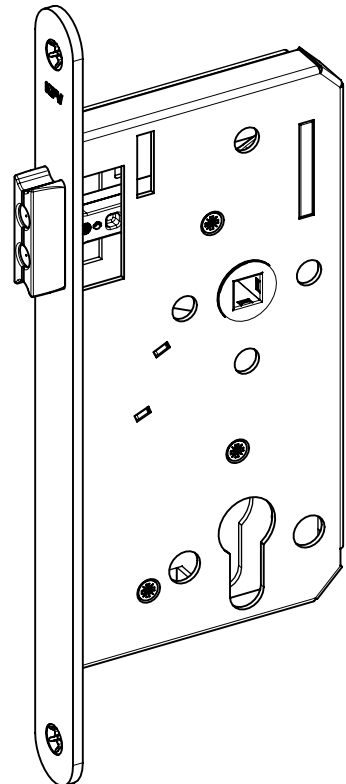
M 1:2
