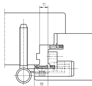
Überschlag 18 mm / Luft 11 mm
