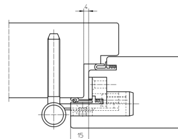
Überschlag 15 mm / Luft 4 mm
