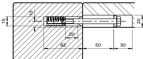
Schnitt B - B Spannschraube
